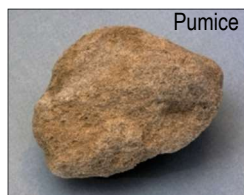
Pumice
